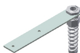
rovný držák pro spirálový kabel, 160x25mm, včetně Spirála žláza M16 (zejména pro rolovací vrata)
